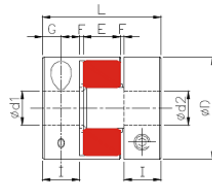
外徑 \phi D20 ~ \phi D30
