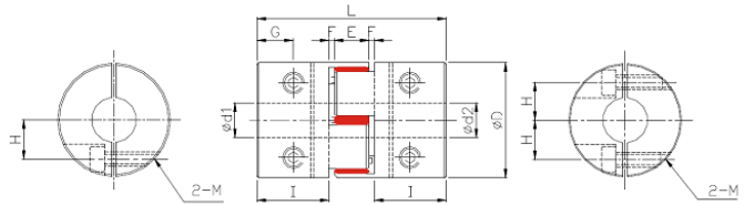
外徑 \phi D40 ~ \phi D65
